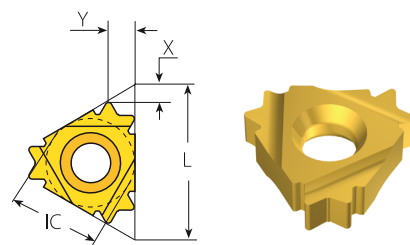
Пластины V6 для внутренней резьбы
