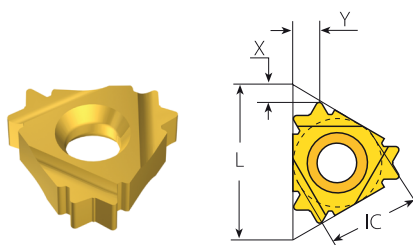
Пластины V6 для наружной резьбы
