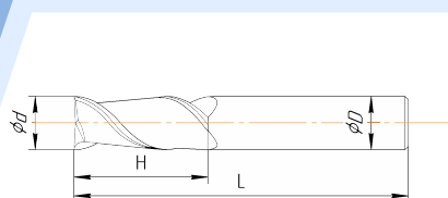
Исполнение 1 d=D
