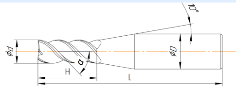
Исполнение 2 d≠D
