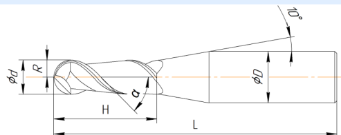
Исполнение 2 d≠D
