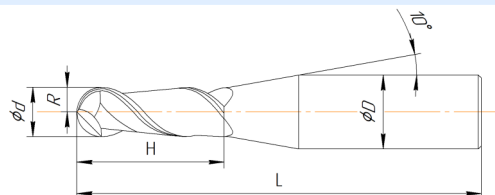
Исполнение 2 d≠D
