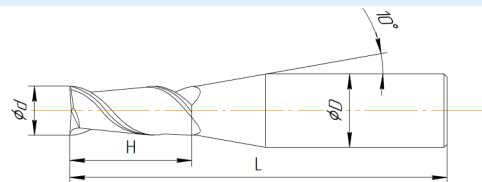
Исполнение 2 d≠D
